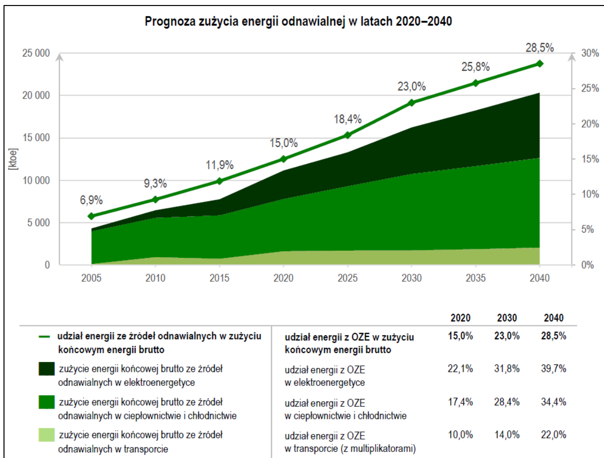
Rysunek 33. Projekcja wzrostu wykorzystania energii odnawialnej w podsektorach, ścieżka wzrostu udziału OZE w końcowym zużyciu energii brutto w perspektywie 2040 r. źródło: Polityka Energetyczna Polski do 2040 r.
